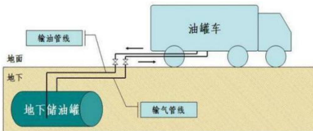
图 2-3 卸油油气回收系统图
