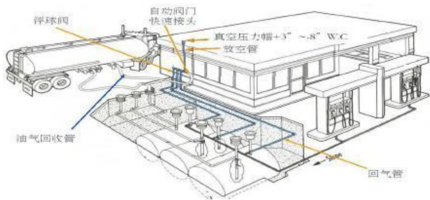
图 4-1 油罐车卸油时油气回收过程示图
