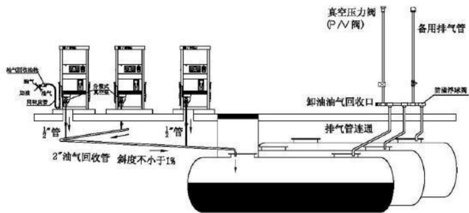
图 4-1 油罐车卸油时油气回收过程示图
