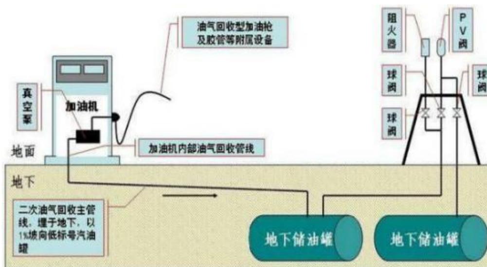
图 2-4 加油油气回收系统图
