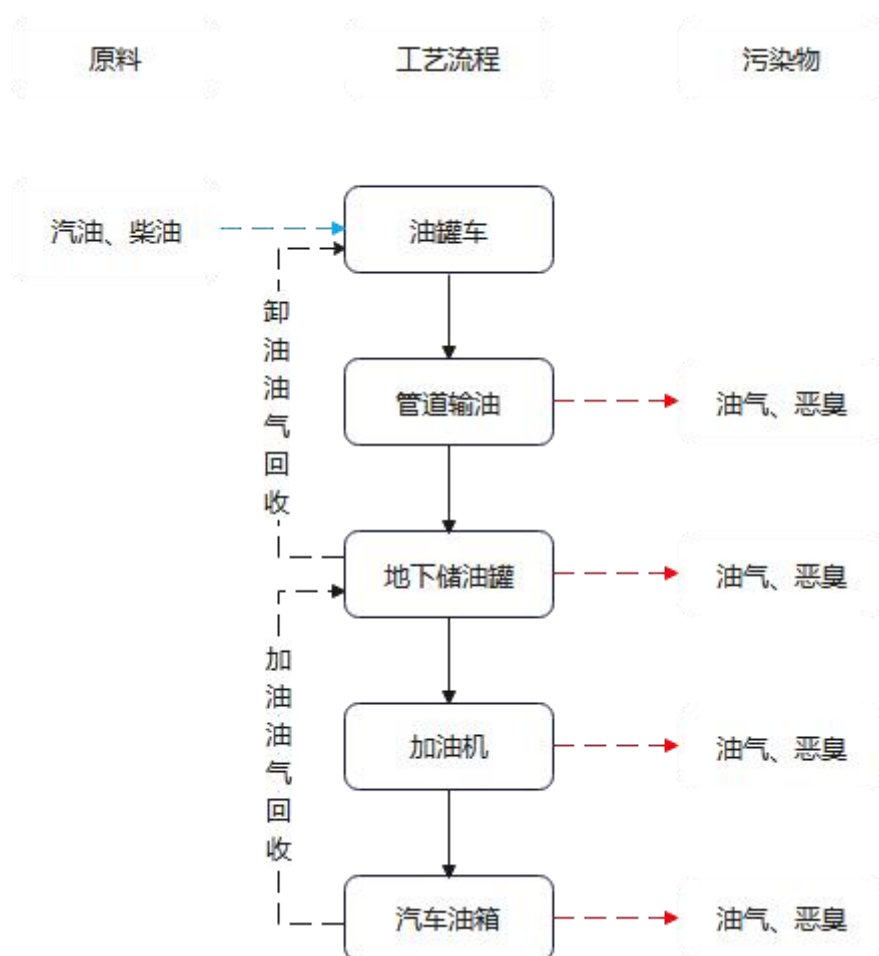
图 2-2 改扩建后加油站运营期工艺流程及产污环节图
