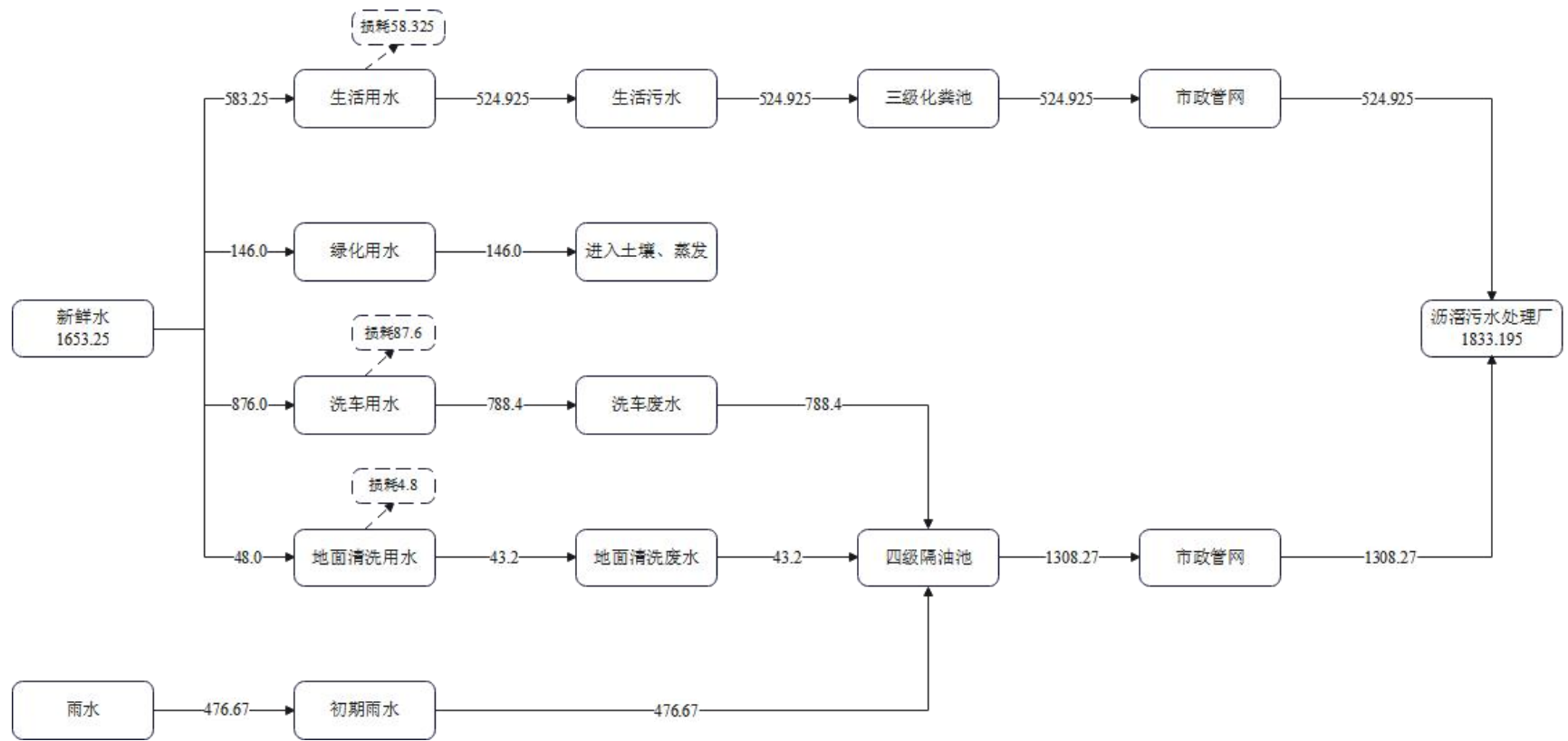
图 2-1 远期水平衡图（单位：m³/a）
