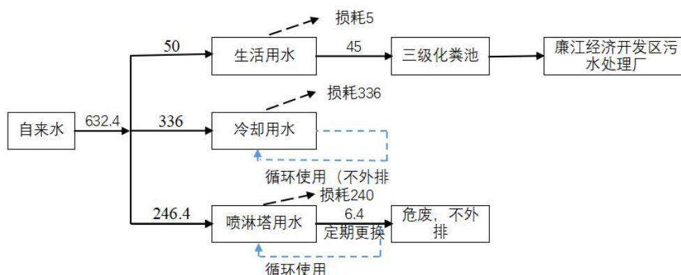
图 2-1 本项目水平衡图（单位：m³/a）
