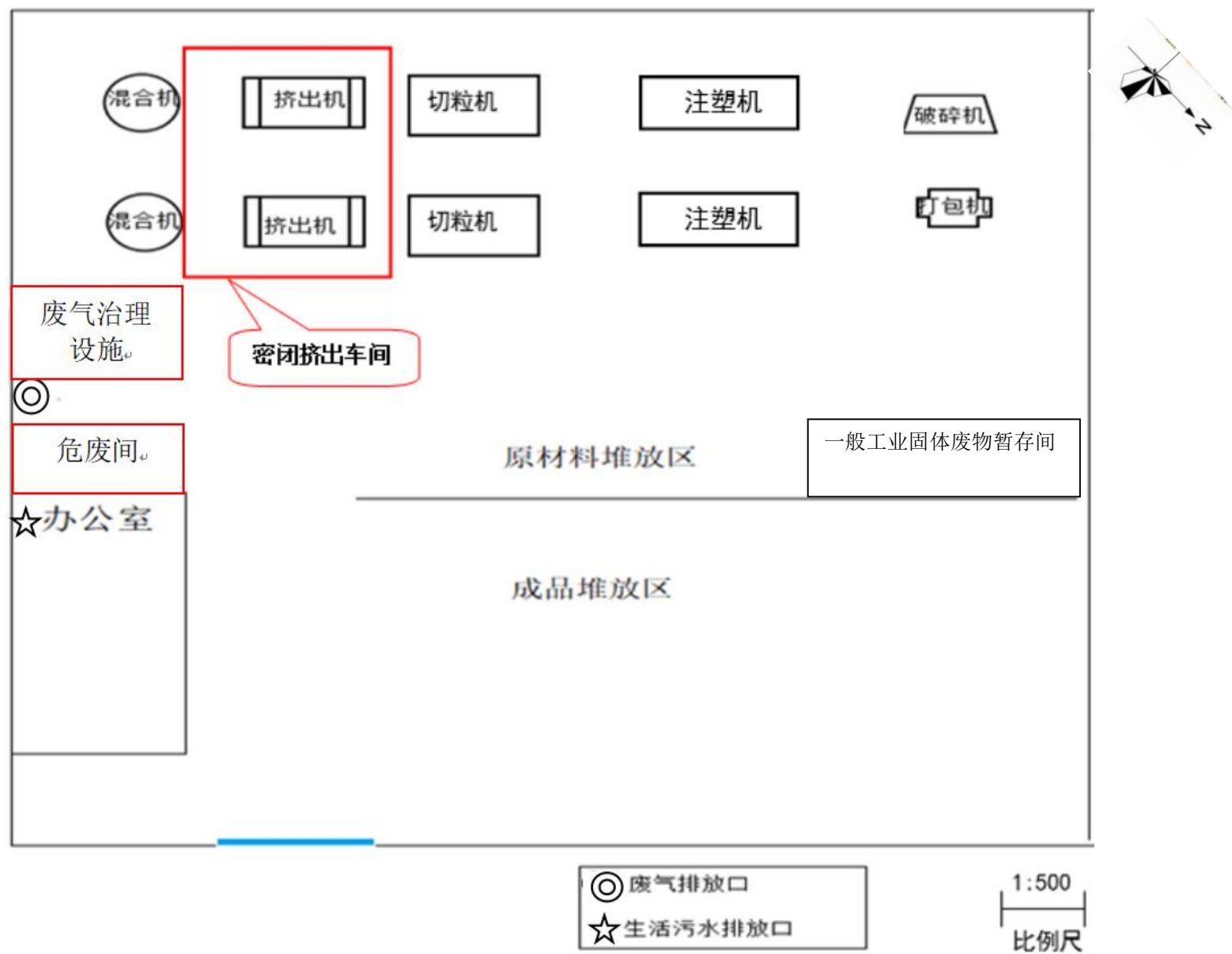
附图 5 项目厂房车间布局图
