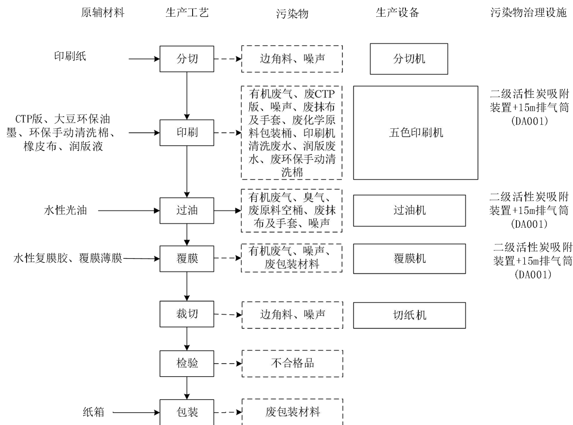
图 2-3 印刷工艺流程及产污环节图
